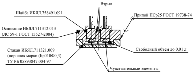
Датчик ИБЯЛ.413226.023-01
