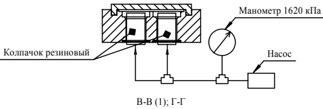
Датчик ИБЯЛ.413226.023-01
